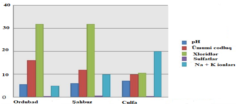
Şəkil 2. Muxtar respublika ərazisindəki dağ çaylarının hidrokimyəvi göstəriciləri
