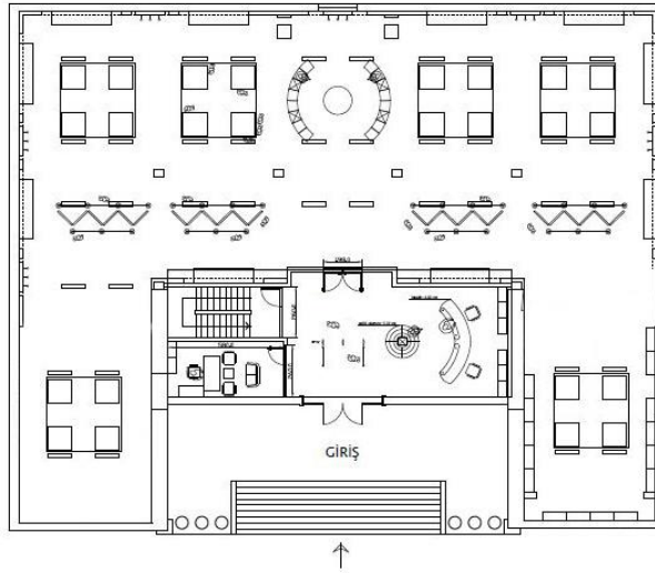
Rəsm 1. Heydər Əliyev adına muzeyin mərtəbə planı
