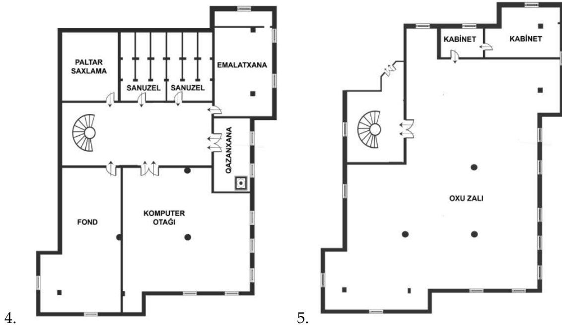
Rəsm 4. Naxçıvan Dövlət Universitetinin Kitabxana binasının zirzəmi qatının planı
